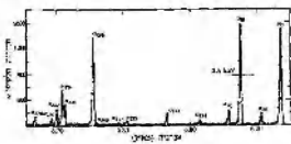
ציר 3. הפקטורים חלקיקי \alpha של {}^{238}_{92}\text{Th} המספרים ליד שיאי ה \alpha וציוריהם את רמת האנרגיה של נרעין התוצר {}^{234}_{90}\text{Ra} שלהם מובילה התפרקות. (מ"ס Engle, ר' ביבל')
